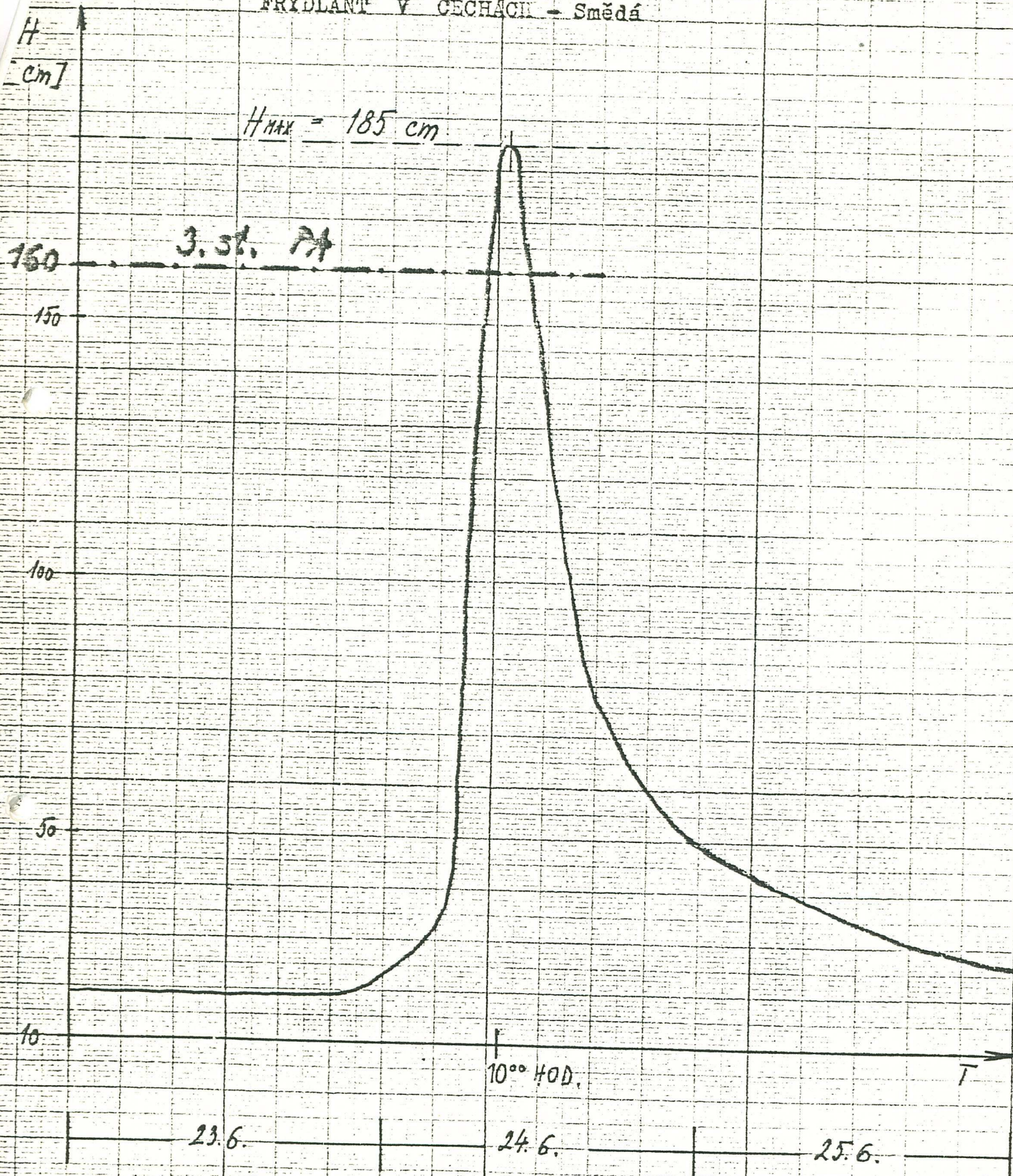
Obr. 7 : Průběh povodňové vlny.
