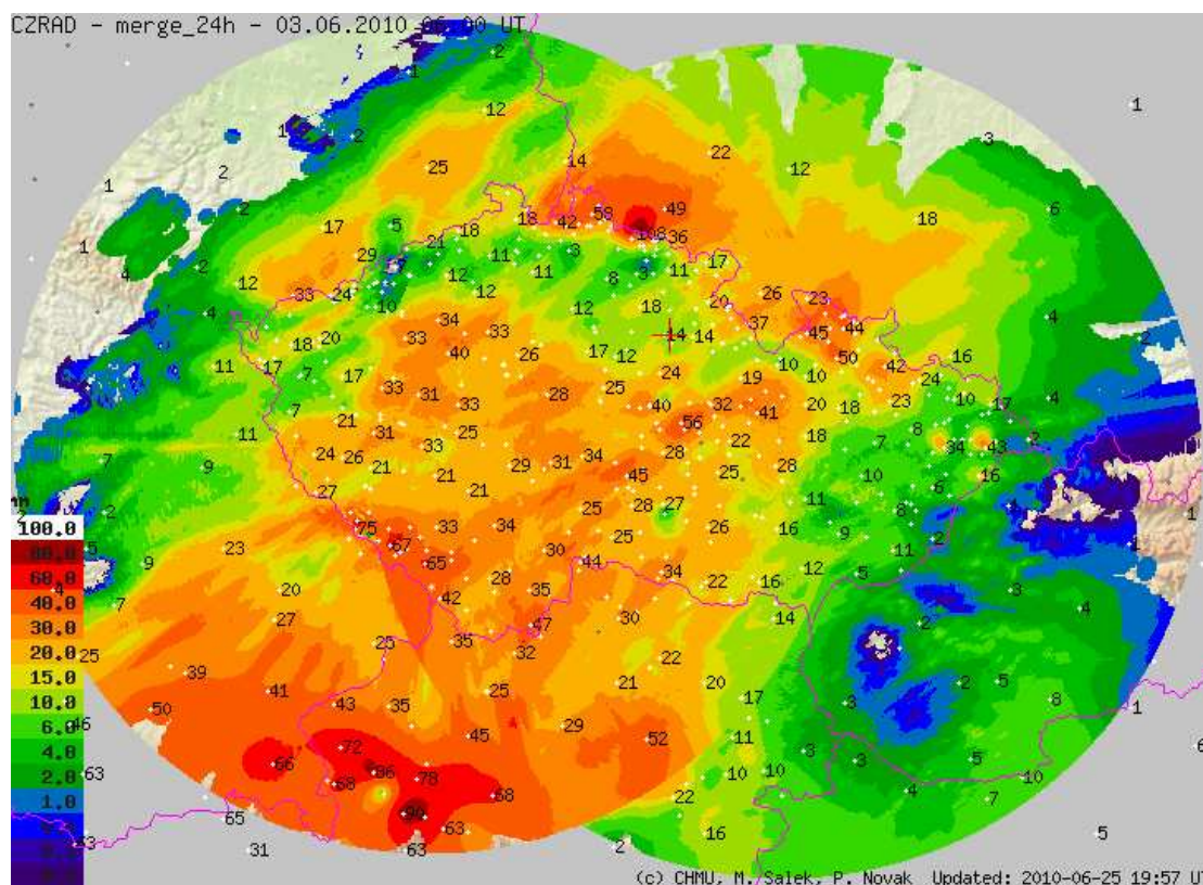
Obr.č.4: KOMBINOVANÝ PLOŠNÝ ODHAD SRÁŽEK RADAR – SRÁŽKOMĚR ZA 24 HODIN DNE 3.6.2010 06:00 UTC
