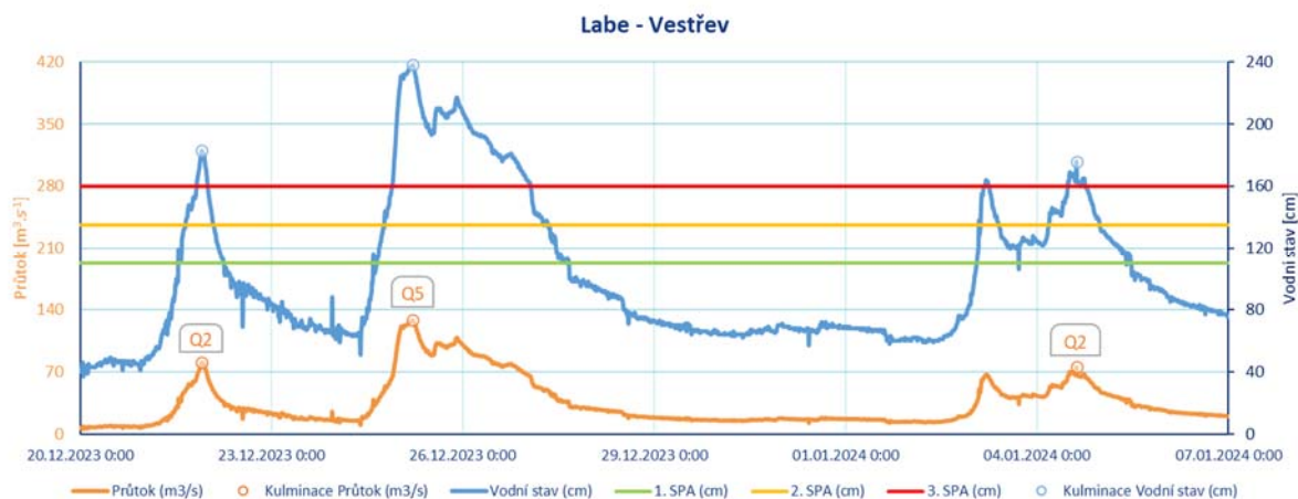
Obr. 2 Průběh průtoků (vodních stavů) na Labi v profilu Vestřev od 20. 12. 2023 do 7. 1. 2024.
