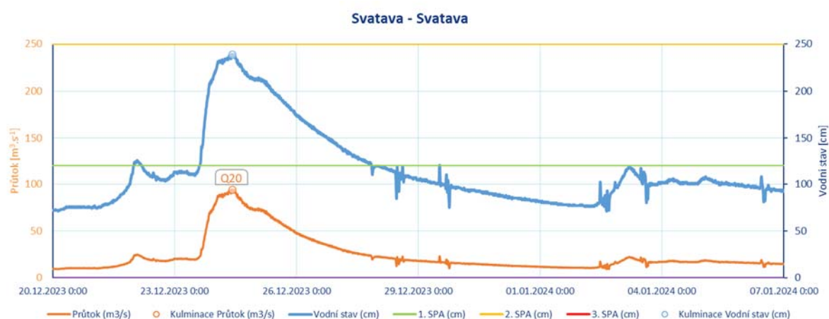
Obr. 33 Průběh průtoků (vodních stavů) na Svatavě v profilu Svataava od 20. 12. 2023 do 7. 1. 2024.
