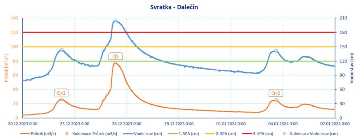
Obr. 43 Průběh průtoků (vodních stavů) na Svratce v profilu Dalečín od 20. 12. 2023 do 7. 1. 2024.
