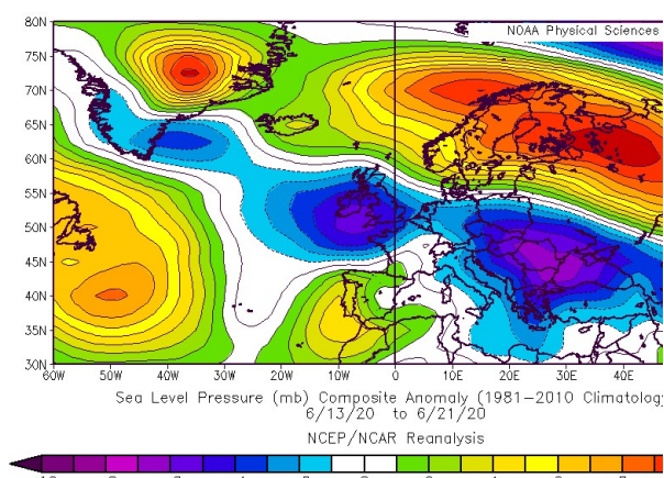
Obrázek 2.1.6 Odchylka od normálu v přízemním tlakovém poli (hPa) v oblasti Atlantik – Evropa v období 13. až 21. června 2020 (normál 1981 – 2010) [2]
