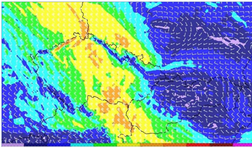
Obrázek 2.4.3 Rozložení směru a rychlosti větru, tedy polohu jet streamu v hladině 925 hPa dne 20. 6. ve 12 UTC na základě modelu Aladin. Pás nejsilnějšího proudění směřoval od severozápadu přímo k oblasti Jizerských hor (oranžový pruh s rychlostmi větru nad 17 m/s) s nejvyššími úhrny srážek. Na obrázku podstatně nižší rychlosti větru od Jizerských hor dále k jihovýchodu (modrý pás) jsou způsobeny tím, že hladina 925 hPa leží pod úrovní hřebenů hor.
