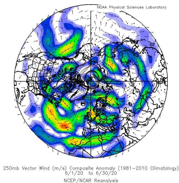
Obrázek 2.1.11 Odchylka od normálu rychlosti větru (m/s) v hladině 250 hPa na severní polokouli za období 1. až 30. června 2020 (normál 1981 – 2010) [2]
