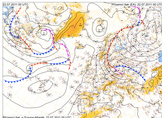
b) 22. 7. 2011 02 SELČ
