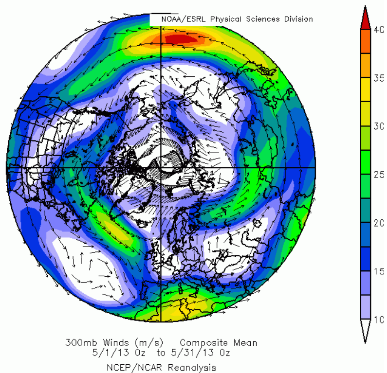
Obr. 1.11 – Průměrný jet stream (300 hPa) v \text{ms}^{-1} na severní polokouli v květnu 2013 (zdroj: NOAA/ESRL).
