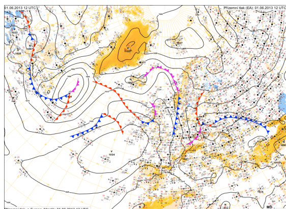
c) 1. 6. 2013 14 SELČ
