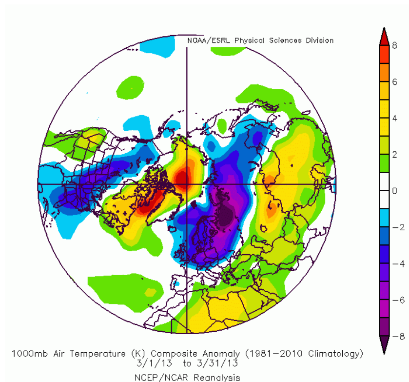
Obr. 1.9: Odchylka teploty vzduchu v 1 000 hPa v °K od normálu (1981–2010) na severní polokouli v březnu 2013 (zdroj: NOAA/ESRL).
