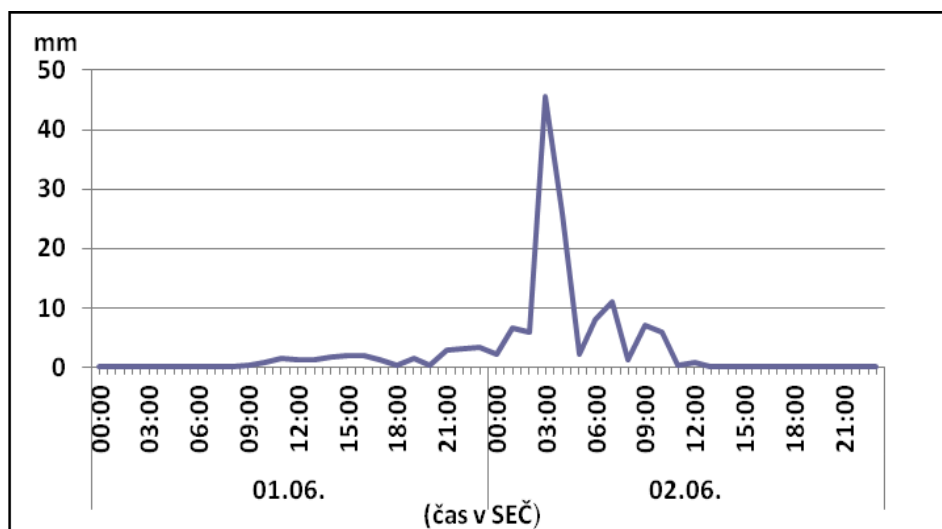
Obr. 2.8a – Průběh hodinových úhrnů srážek na stanici Horní Maršov (povodí Úpy) od 1. 6. 01 SELČ do 3. 6. 2013 00 SELČ.
