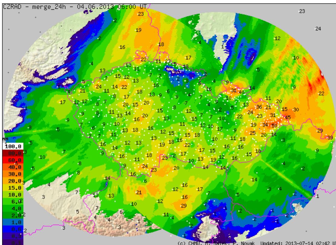
Obr. 1.28 – Množství spadlých srážek za období od 3. 6. 08 SELČ do 4. 6. 2013 08 SELČ kombinací radarových odhadu a měření ze srážkoměrů.
