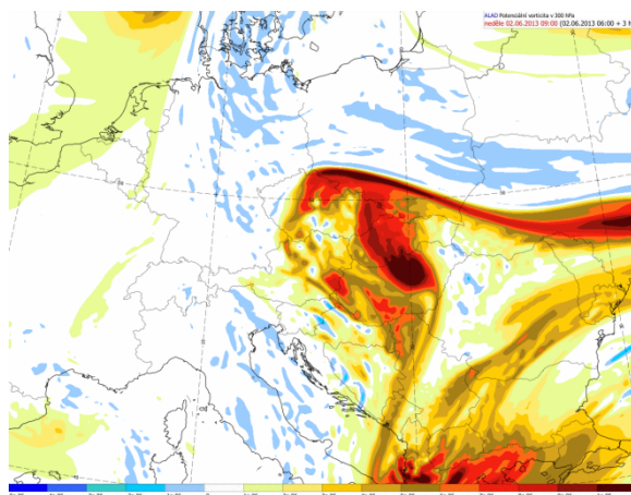
a) Potenciální vorticitu (PV) v hladině 300 hPa.
