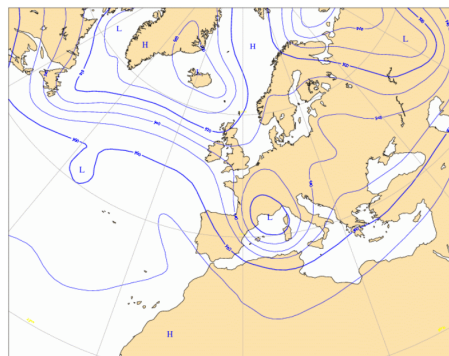
b) 11. 8. 2002 02 SELČ
