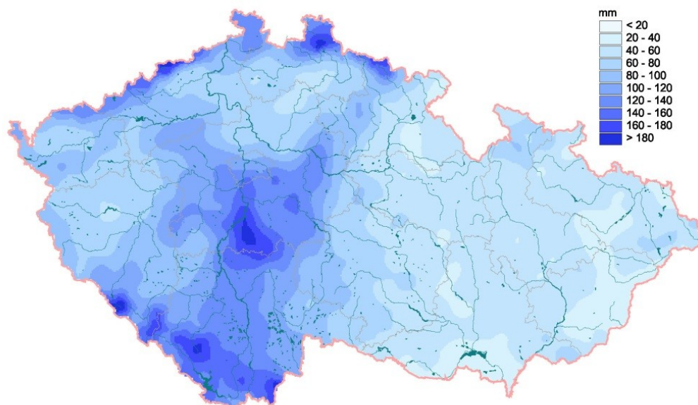
Obr. 2.7 – Úhrn srážek od 29. 5. 08 SELČ do 3. 6. 2013 08 SELČ na území ČR.
