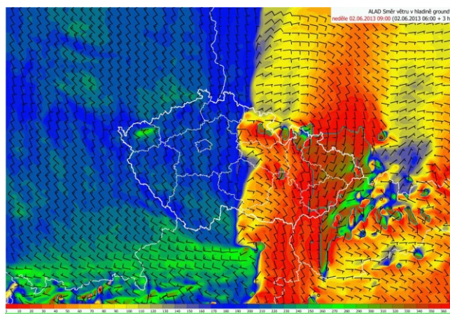
b) Přizemní konvergence vzduchu (barevné zobrazení směru větru).
