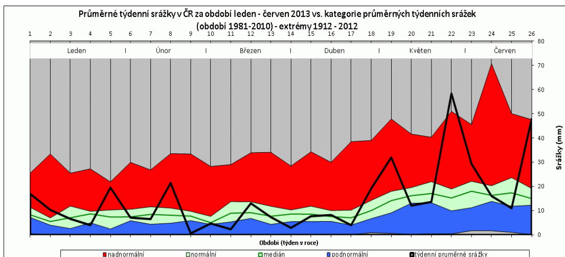
Obr. 1.2 – Průměrné týdenní srážky v ČR za období leden až červen 2013 v porovnání s dlouhodobými hodnotami (srovnávací období 1981–2010, extrémy za období 1912–2012).
