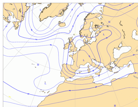
d) 30. 5. 2013 02 SELČ
