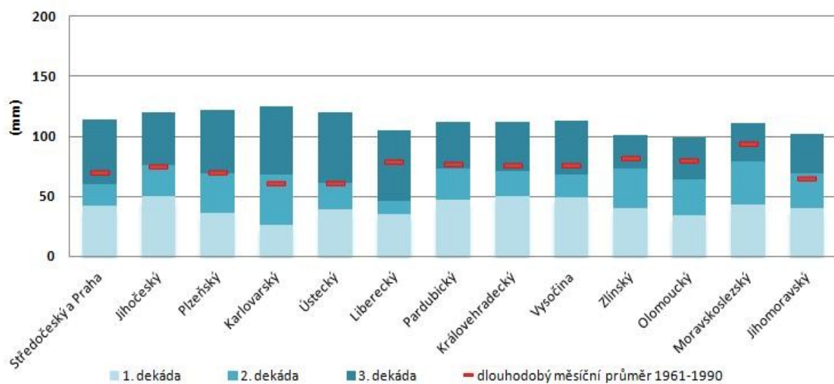
Obr. 2.3 – Průměrné úhrny srážek [mm] v krajích ČR v květnu 2013 po dekádách.
