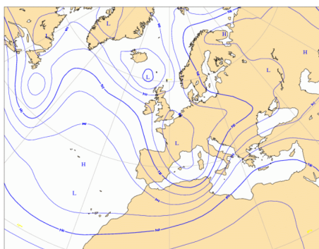
c) 15. 5. 2010 02 SELČ
