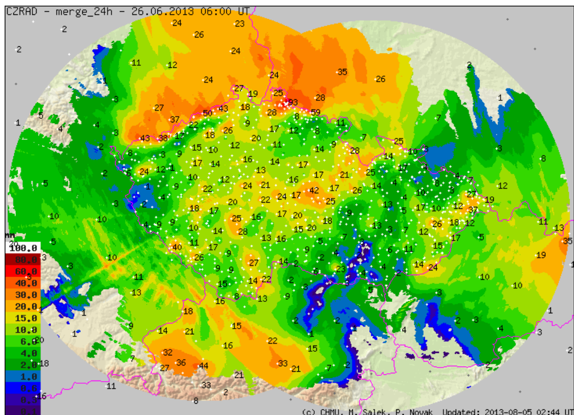
Obr. 1.41 – Množství spadlých srážek za období od 25. 6. 08 SELČ do 26. 6. 2013 08 SELČ kombinací radarových odhadu a měření ze srážkoměrů.
