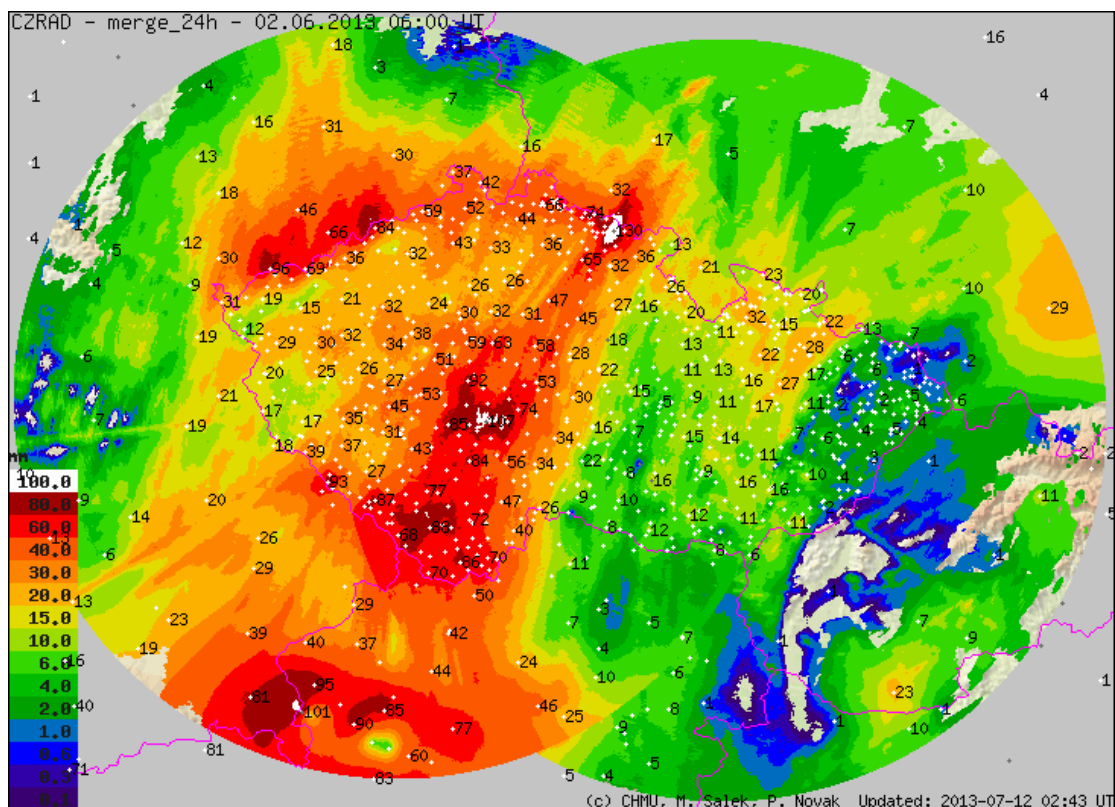
Obr. 1.26 – Množství spadlých srážek za období od 1. 6. 08 SELČ do 2. 6. 2013 08 SELČ kombinací radarových odhadu a měření ze srážkoměrů.
