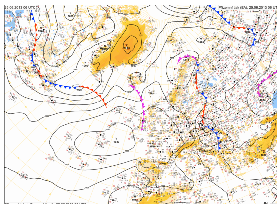
d) 25. 6. 2013 08 SELČ
