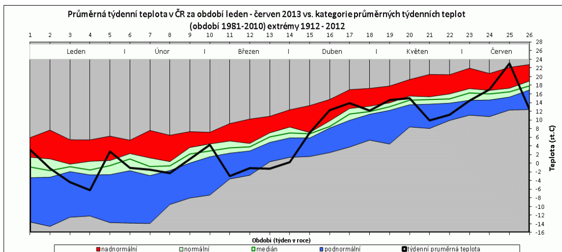
Obr. 1.1 – Průměrná týdenní teplota v ČR za období leden až červen 2013 v porovnání s dlouhodobými hodnotami (srovnávací období 1981–2010, extrémy za období 1912–2012).
